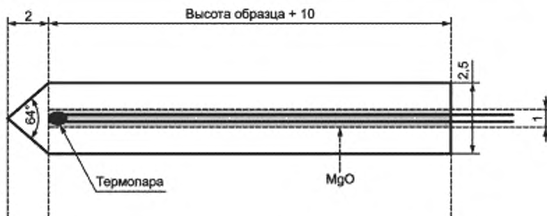
Рисунок 1 — Схематичное изображение испытательного гвоздя
