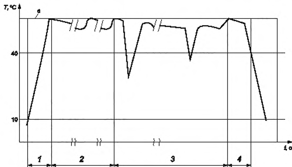
1 — этап С: период заполнения и нагрева (см. 7.7); 2 — этап D: подвод мощности в режиме ожидания (см. 7.8); 3 — этап E: отбор воды (см. 7.9), 4 — этап F: смешанная вода при температуре 40 °С и эталонная температура горячей воды (см. 7.10). T — температура, °С; t — время, с; a — заданная температура
