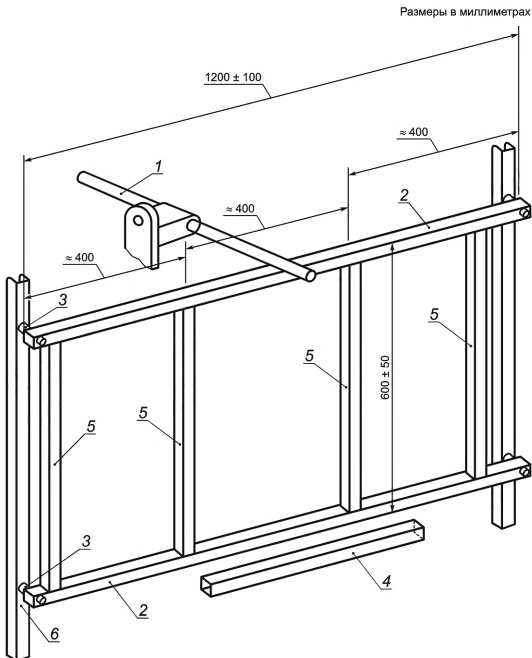
1 — ударное устройство; 2 — стальная лестница; 3 — резиновая втулка; 4 — газовая горелка ленточного типа; 5 — неподвижный вертикальный элемент; 6 — опора лестницы
