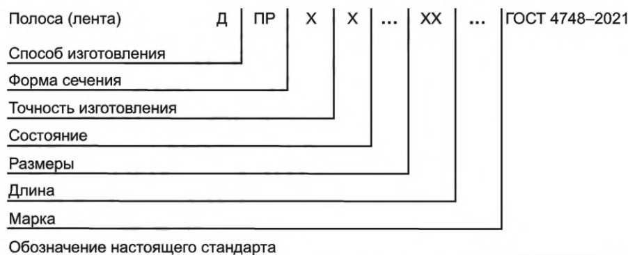
Рисунок 1 — Схема условного обозначения полос и лент
