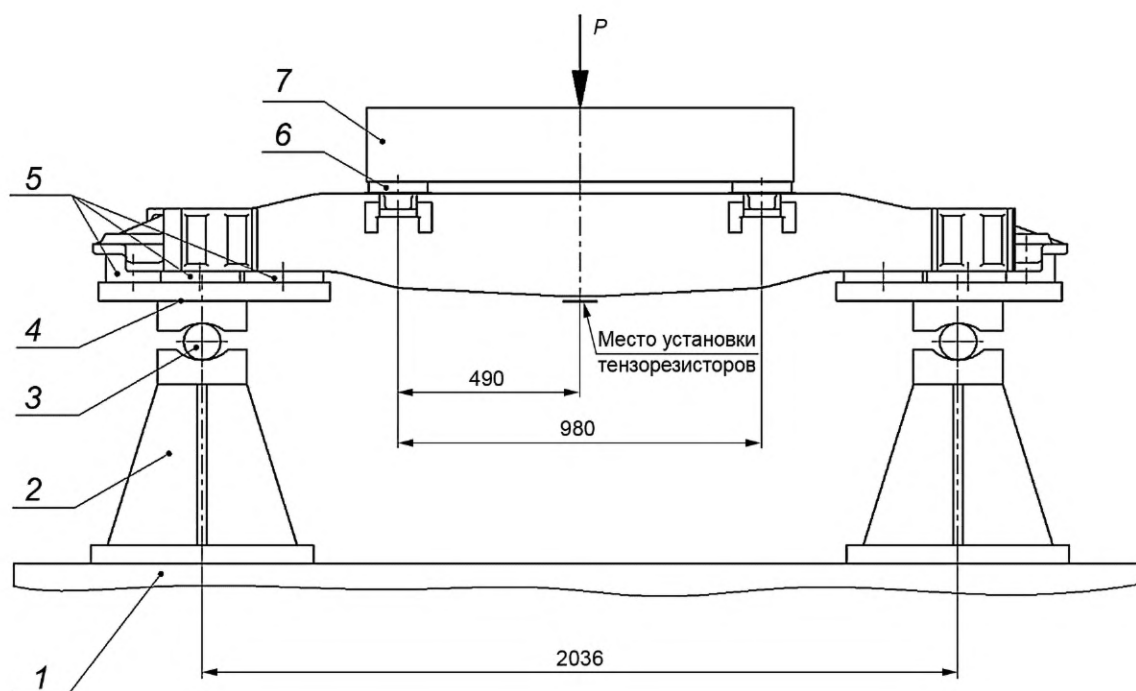
1 — стол испытательного стенда; 2 — опорная тумба; 3 — цилиндр; 4 — опорный элемент с фасонной плитой; 5, 6 — сегменты; 7 — брус
