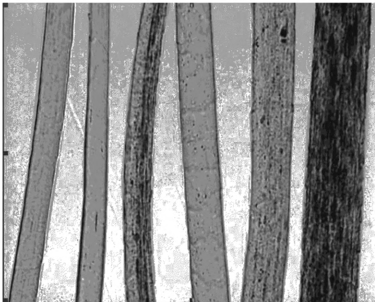
Рисунок С.22 — Изображение волокон, чешуйки которых неотчетливо видны и вызывают сомнения
