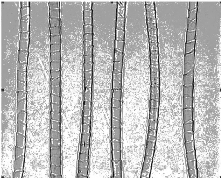
Рисунок С.11 — Изображение волокон с чешуйками венчикообразной формы с очень высокой частотой, имеющих характеристики тонкой овечьей шерсти
