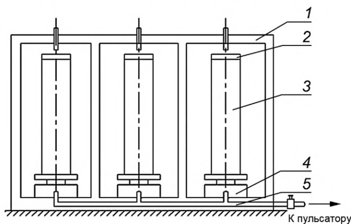
Рисунок 1 — Схема испытательной машины для одновременного испытания трех образцов
