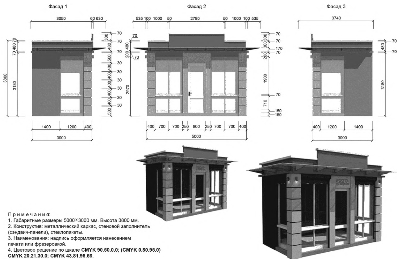
Рисунок А.10 — Павильон 5×3 м
