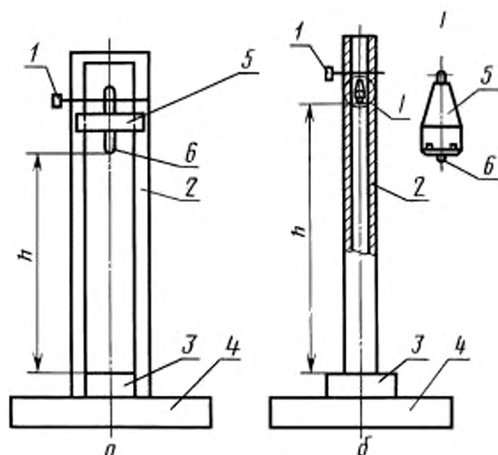
1 — стопор; 2 — направляющее устройство; 3 — испытуемый образец; 4 — основание; 5 — груз; 6 — шарик диаметром 25 мм
