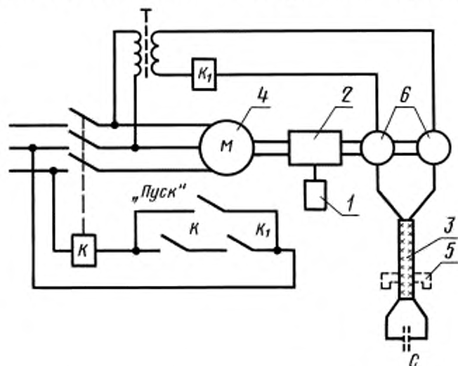
1 — счетчик; 2 — редуктор; 3 — испытуемый шнур; 4 — электродвигатель; 5 — груз; 6 — токоъемные кольца
