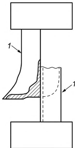
Рисунок D.2 — Зажим испытуемых проб в губках зажима
