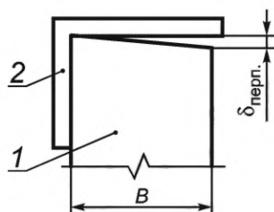
1 — панель; 2 — поверочный угольник 90^\circ ; B — ширина панели
