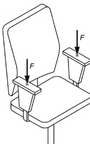
Рисунок 29 — Испытание подлокотников под действием направленной вниз статической нагрузки — по центру подлокотников
