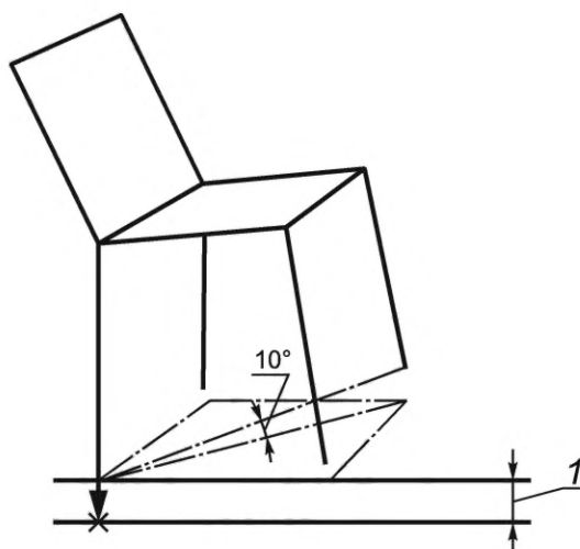
Рисунок 24 — Испытание на удар при падении с высоты стола
