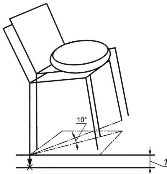
Рисунок 23 — Испытание на удар при падении штабелируемой мебели для сидения
