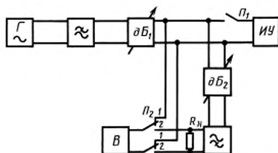
Г — измерительный генератор; ⊗ — фильтр нижних частот; дБ 1 , дБ 2 — магазины затуханий; ⊗ — фильтр верхних частот; В — избирательный измерительный прибор; ИУ — измеритель уровня; П — переключатель; R н — нагрузка фильтра
