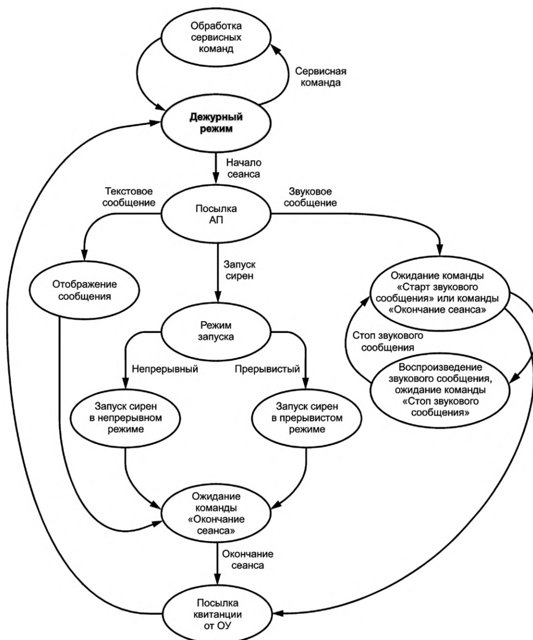
Рисунок Б.1 — Графы состояний устройства управления
