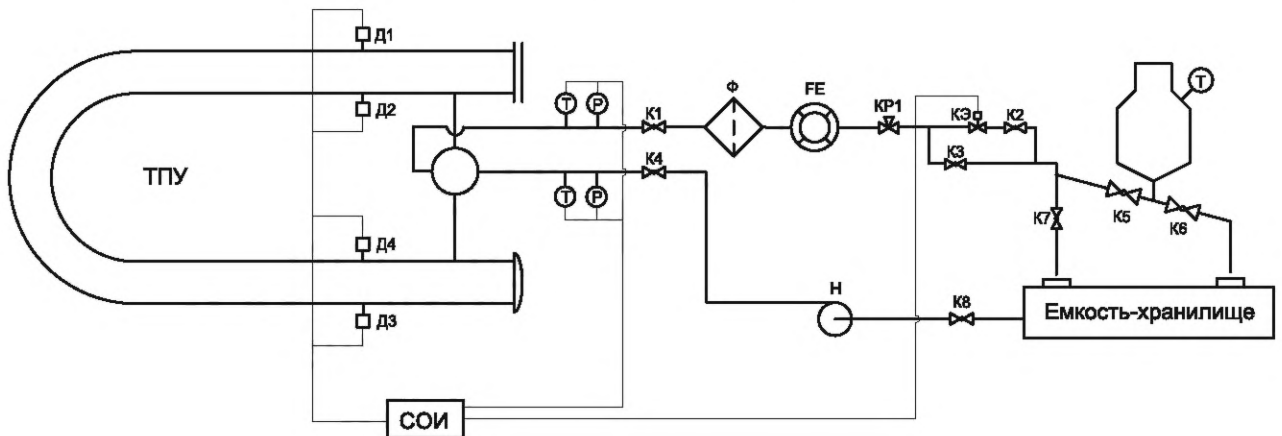
Рисунок А.4.1 — Схема монтажа ТПУ и ПУ с мерником (с нижним заполнением) с электромагнитным клапаном в качестве переключателя потока (с остановкой поршня)
