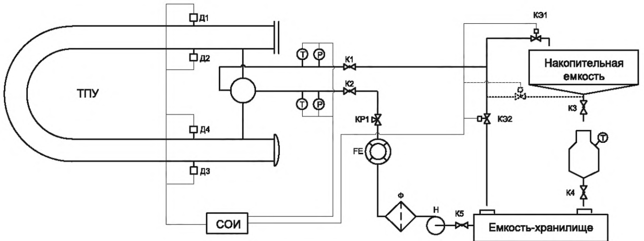
Рисунок А.3.2 — Схема монтажа ТПУ и ПУ с ВУ с электромагнитными клапанами в качестве переключателя потока
