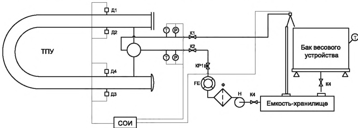
Рисунок А.2.1 — Схема монтажа ТПУ и ПУ с ВУ с перекидным устройством в качестве переключателя потока
