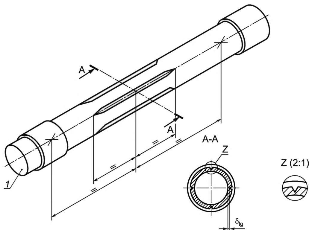
1 — концевая заглушка; \delta_{lg} — остаточная толщина, соответствующая 0,78—0,82 номинальной толщины стенки испытуемой трубы, мм
