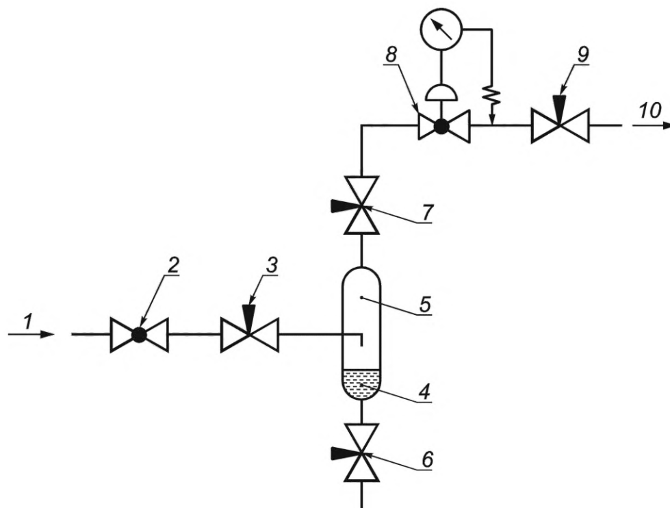
1 — исследуемый газ из газопровода; 2 — шаровой кран; 3, 7, 9 — вентили; 4 — конденсат; 5 — коллекторная емкость; 6 — продувочный вентиль; 8 — редуктор давления (при необходимости); 10 — исследуемый газ на анализ
