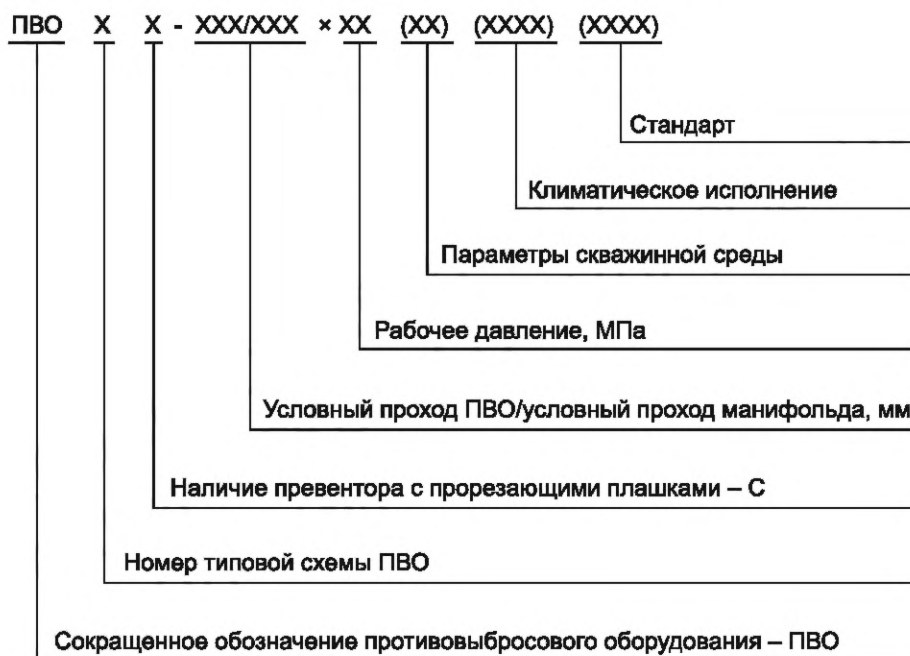
Рисунок 1 — Структура условного обозначения ПВО
