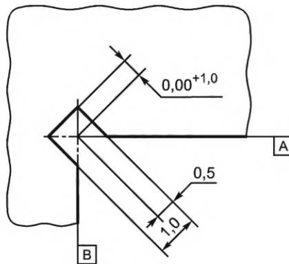
Рисунок Б.5 — Деталь А (размеры подреза)
