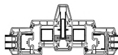
в) Торцевое соединение коробок с использованием фасадного соединителя (с возможностью компенсации температурных деформаций)
