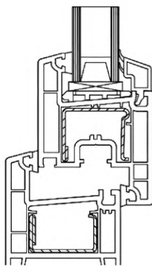
а) Оконный блок из трехкамерных профилей
