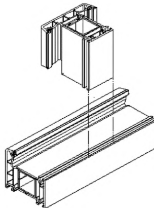
д) Сварка под углом 90°
