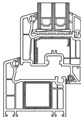
в) Оконный блок из пятикамерных профилей
