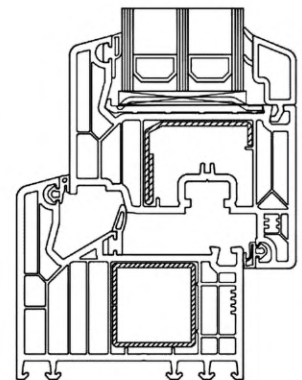
г) Оконный блок со створкой из шестикамерного и коробкой из семикамерного профилей
