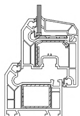
и) Балконный дверной блок из четырехкамерных профилей с поворотным и поворотно-откидным открыванием створки
