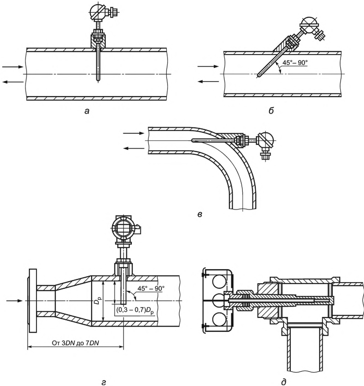
Рисунок 3 — Схема расположения чувствительного элемента преобразователя температуры
