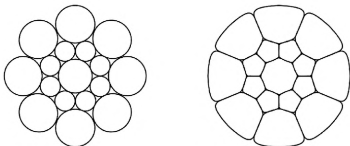
а) Прясть до уплотнения
