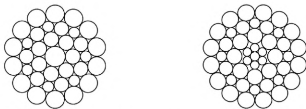
а) Прядь с одной центральной проволокой
