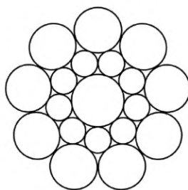
Рисунок 6 — Конструкция «Сил»
