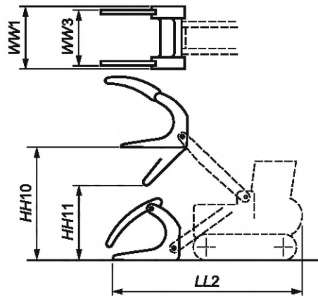
Рисунок 23 — Размеры рабочего оборудования и челюстного захвата, установленных на погрузчики
