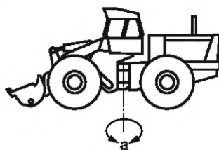
Рисунок 8 — Шарнирно-сочлененная рама
