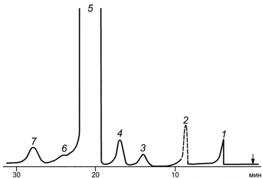
1 — пиридин; 2 — додекан (внутренний эталон); 3 — фенол; 4 — анилин; 5 — о-крезол; 6 — м + п-крезолы; 7 — 2,6-ксиленол
