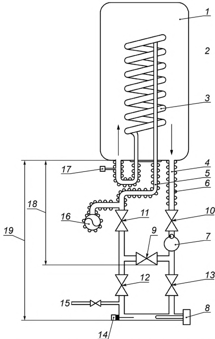
1 — испытуемый бак; 2 — место измерения температуры окружающего воздуха; 3 — нагревательная спираль; 4, 5 — место измерения температуры; 6 — изоляция; 7 — насос; 8 — электрический нагреватель; 9 — кран 1; 10 — кран 2; 11 — кран 3; 12 — кран 4; 13 — кран 5; 14 — водяной термостат; 15 — подпитка; 16 — изолированный расширительный бачок; 17 — регулирующий вентиль; 18 — короткий контур; 19 — длинный контур
