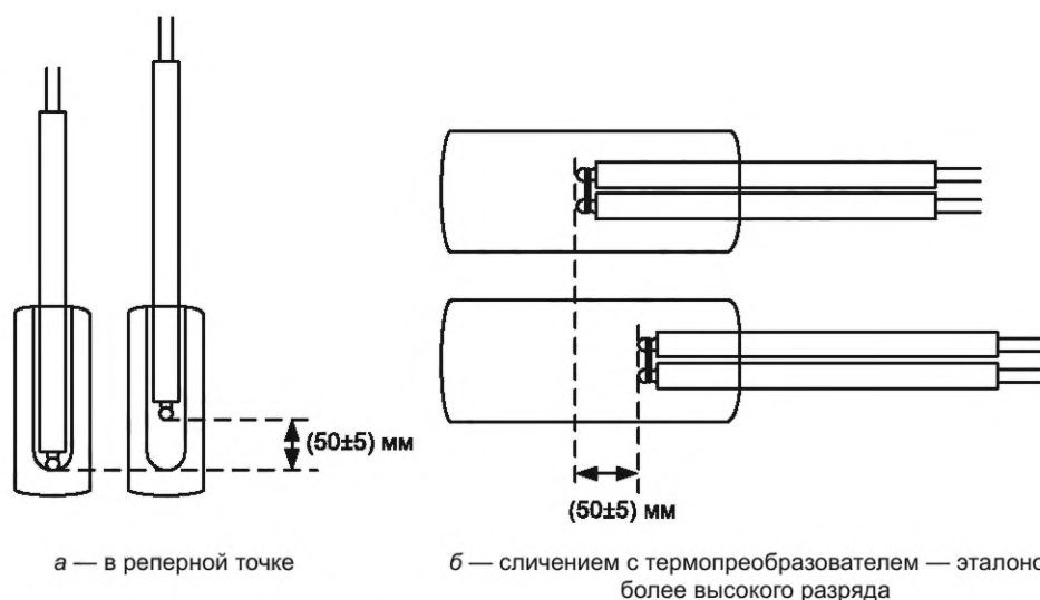
Рисунок 2 — Схема размещения термомпреобразователей при определении неоднородности
