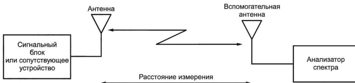
Рисунок 3 — Блок-схема измерительной установки для измерения мощности в неактивном режиме изделия со встроенными антеннами
