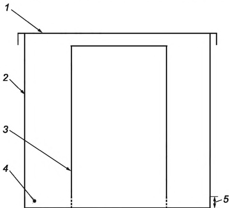
1 — куполообразная крышка; 2 — кристаллизатор или другая емкость; 3 — корковая пробка; 4 — окрашенный раствор; 5 — высота 3 мм (6 мм для пробок со снятой фаской)
