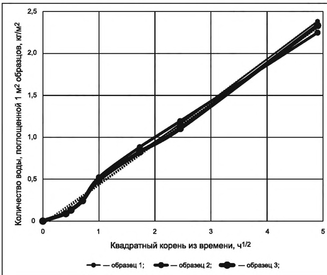
Рисунок А.1 — График капиллярного всасывания воды в радиальном направлении образцами из термически модифицированной древесины дуба
