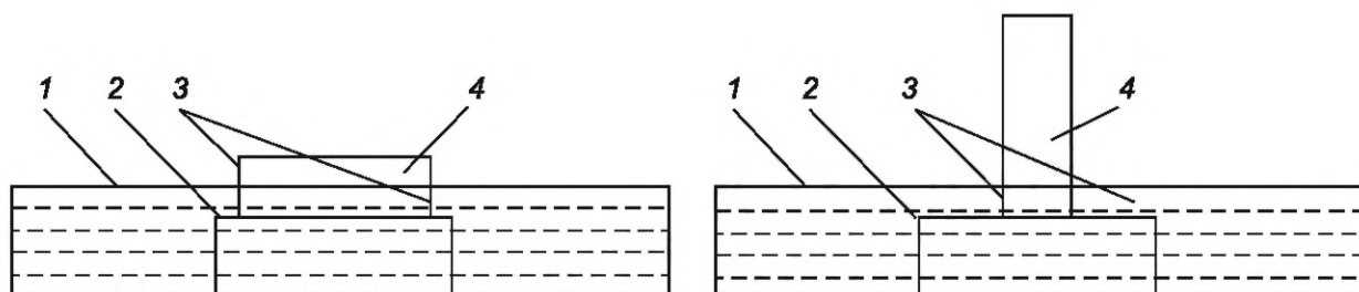
а) Капиллярное всасывание в радиальном и тангенциальном направлениях
