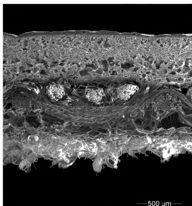
Рисунок А.12 — Сечение полимерного материала, дублированного с кожевными волокнами
