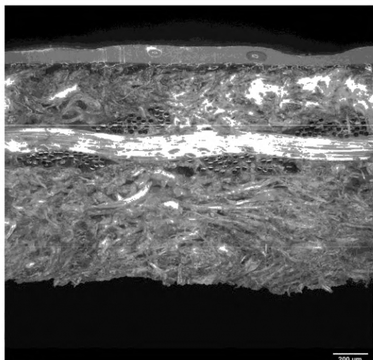
Рисунок В.11 — Сечение текстильного материала, покрытого коженными волокнами
