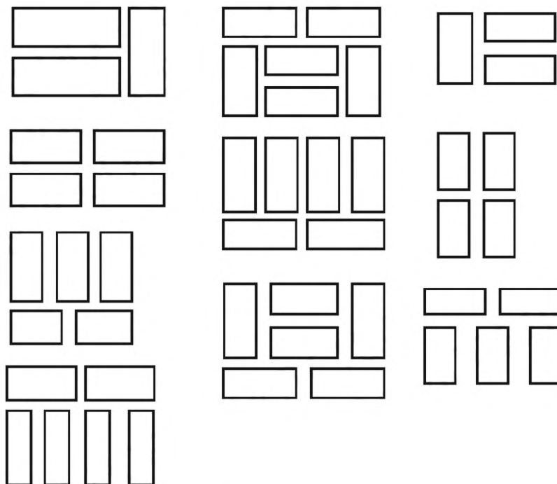
Рисунок А.1 — Рядовая укладка
