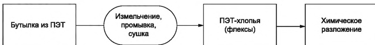
Рисунок А.1 — Предварительная обработка [получение ПЭТ-хлопьев (флекссы)]
