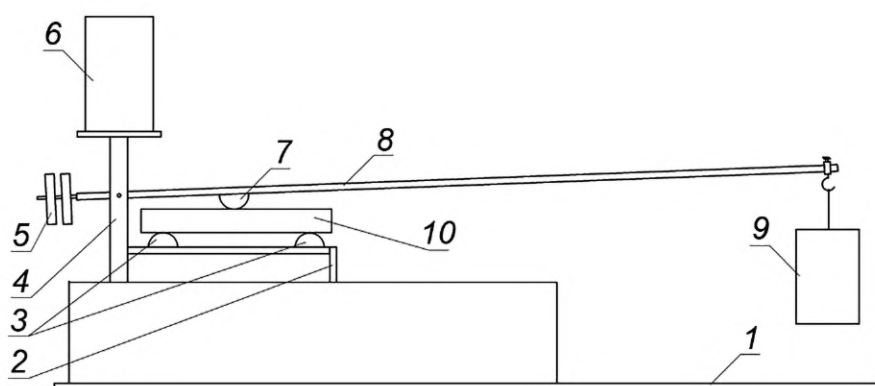
Рисунок 1 — Устройство для формирования образцов
