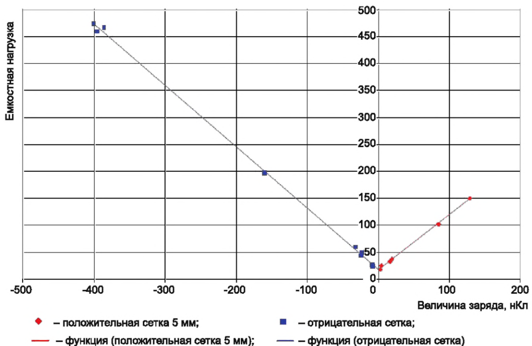
Рисунок D.4 — Пример зависимости емкостной нагрузки от величины коронного заряда
