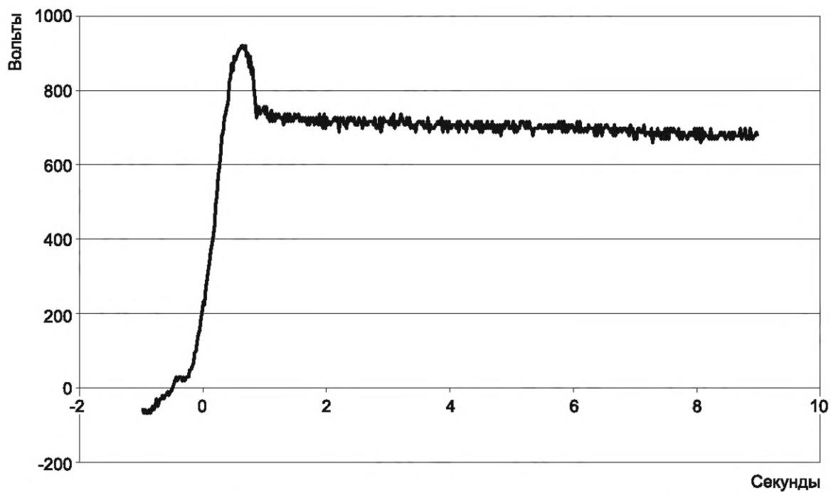
Рисунок В.2б — Электрическое напряжение тела, измеренное во время вставания с сиденья поочередно каждой ногой
