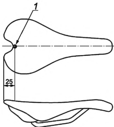
1 — точка нагружения
