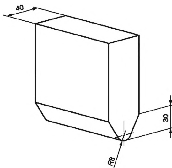
Рисунок 24 — Размеры ударника
