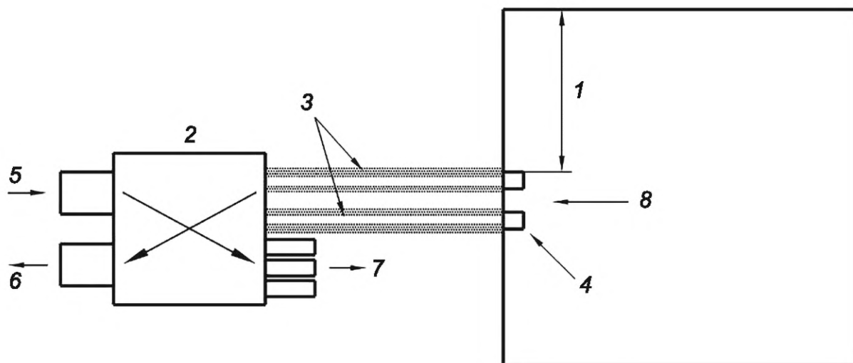
1 — минимальное расстояние в 1 м (от всех поверхностей); 2 — испытуемый агрегат; 3 — звукоизолированные жесткие воздуховоды 1,5 м; 4 — испытуемые соединения воздуховодов; 5 — приточный воздух; 6 — удаляемый воздух; 7 — выход приточного воздуха (три выхода); 8 — вытяжки (два выхода одинакового диаметра)
