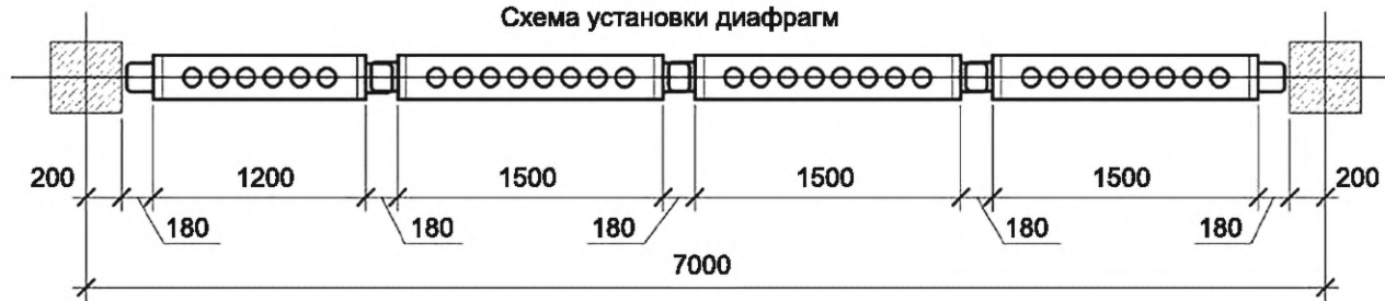
Схема установки диафрагм
