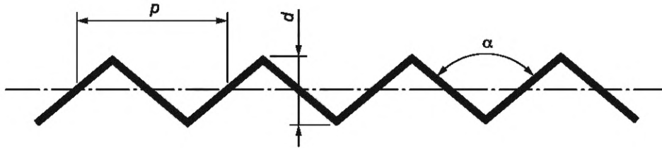
Рисунок 2 — Треугольный профиль
