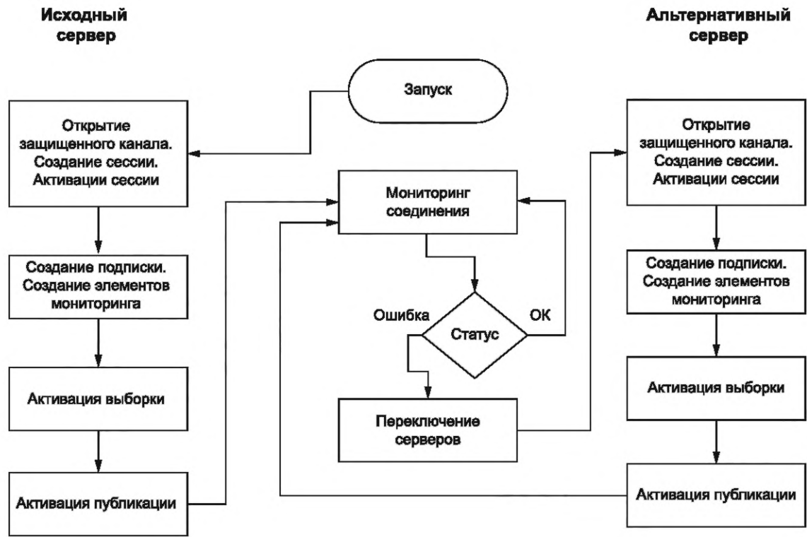
Рисунок 29 — Холодное переключение
