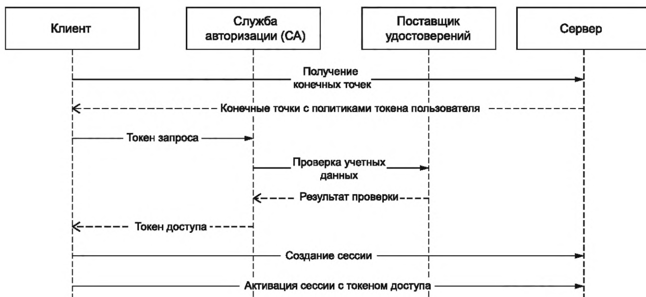
Рисунок 24 — «Косвенное рукопожатие» с поставщиком удостоверений
