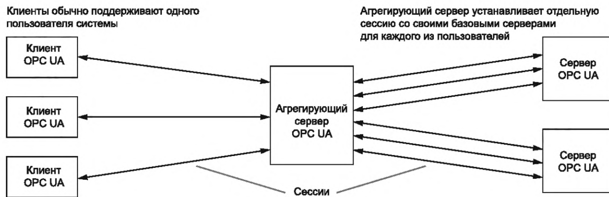
Рисунок 14 — Мультиплексирование пользователей в сессии
