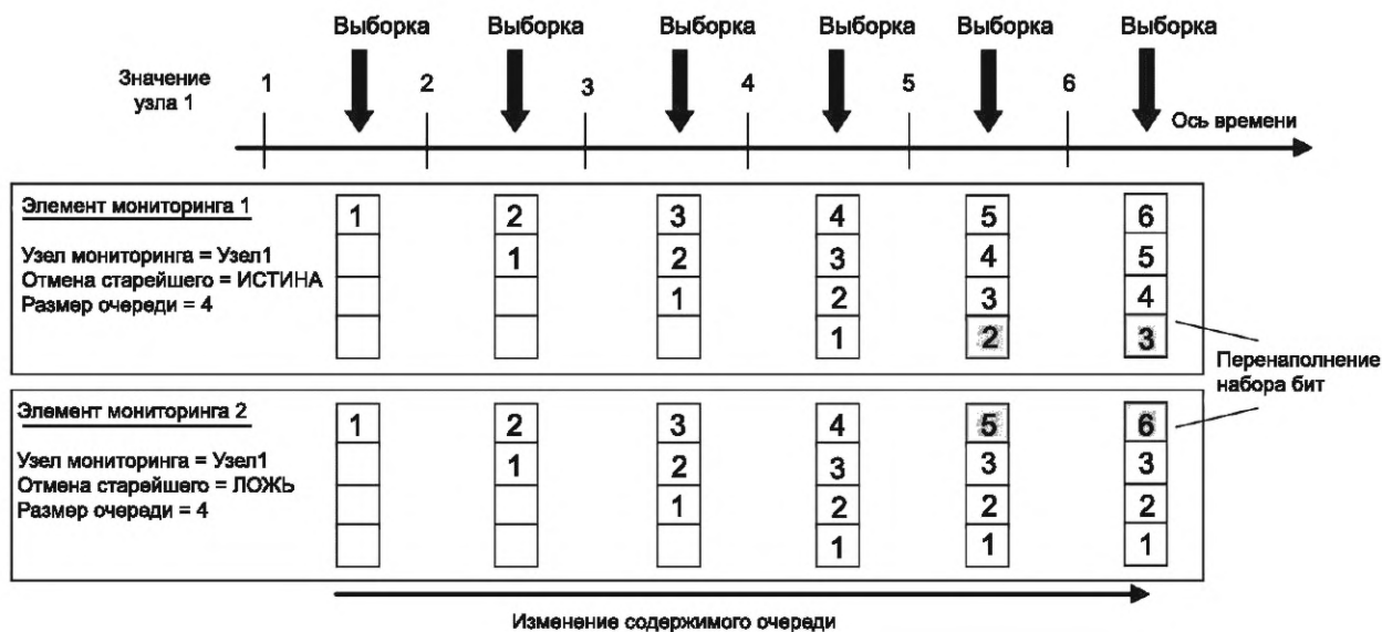
Рисунок 17 — Обработка переполнения очереди
