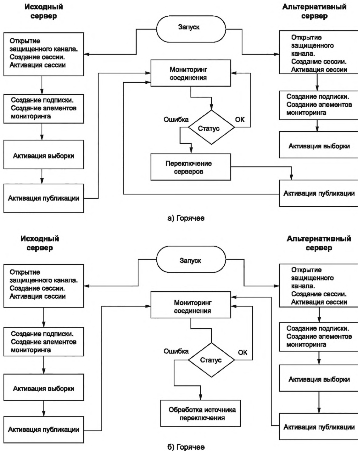
Рисунок 31 — Автоматическое переключение
