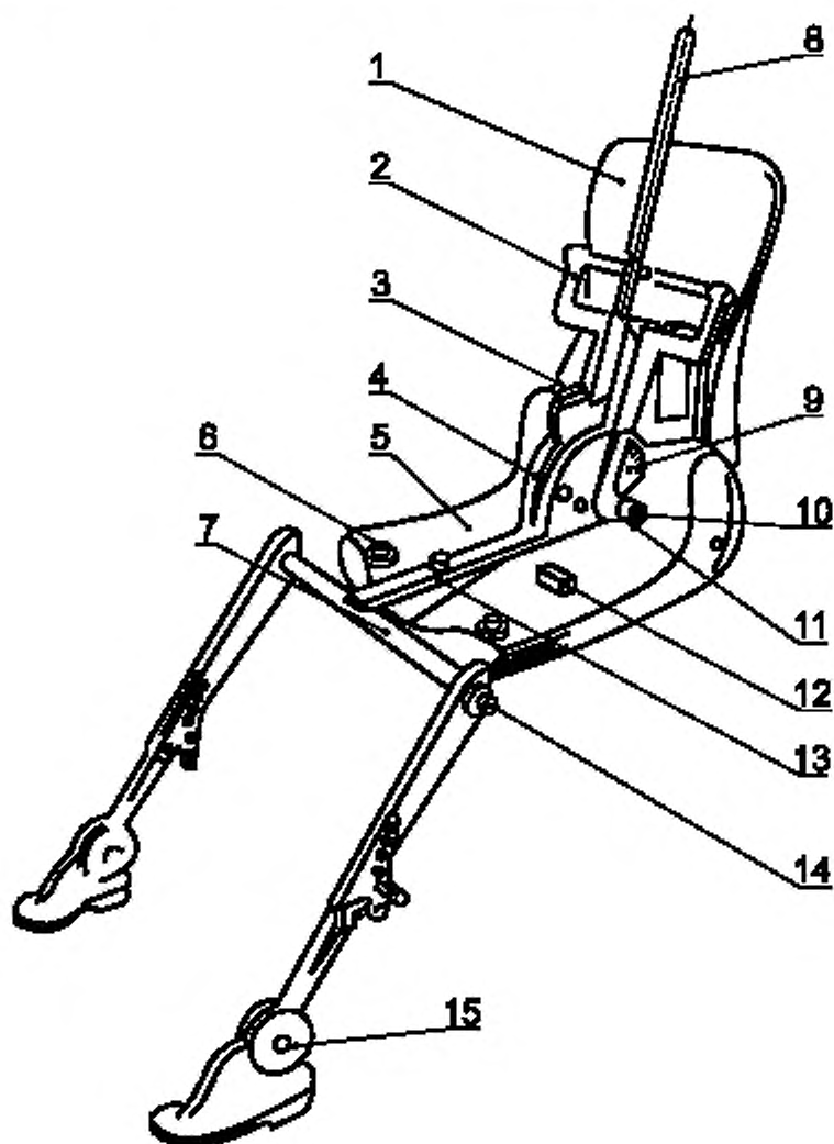
1 — спинка; 2 — кронштейн спинных грузов; 3 — уровень угла наклона спинки; 4 — круговой сектор наклона бедра; 5 — основание; 6 — кронштейн набедренных грузов; 7 — коленный шарнир T ; 8 — штырь; 9 — круговой сектор наклона спинки; 10 — визирные метки точки H ; 11 — ось вращения точки H ; 12 — поперечный уровень; 13 — кронштейн бедра; 14 — круговой сектор сгиба колена; 15 — круговой сектор сгиба ступени
