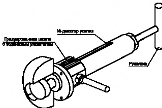
Рисунок 5.1 — Приспособление для измерения выступов
