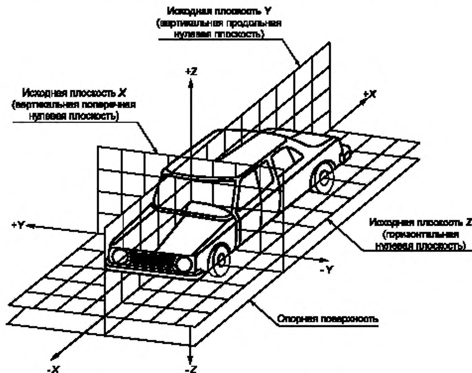
Рисунок 7.3 — Трехмерная система координат
