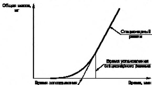
Рисунок 4 — Общий вид графика изменения общей массы протифундировавшей испытательной жидкости во времени
