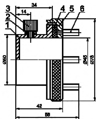
Рисунок 3 — Диффузионная ячейка для испытания гравиметрическим методом
