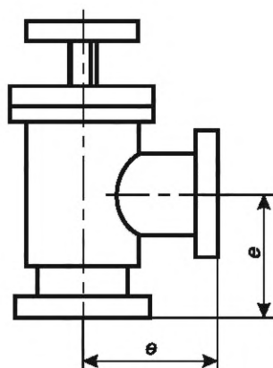
Рисунок 1 — Угловой клапан
