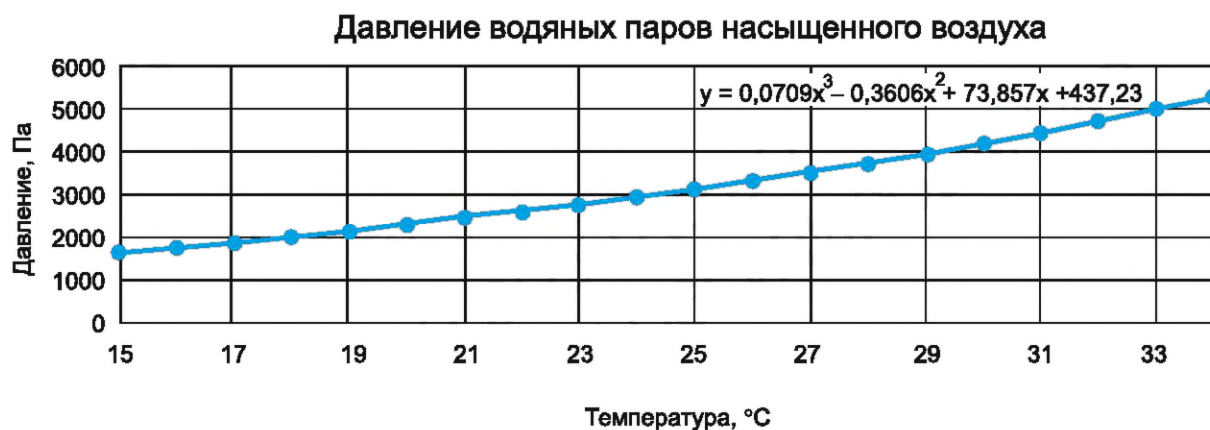
Рисунок 1 — График зависимости давления водяных паров насыщенного воздуха от температуры на основании данных таблицы 5
