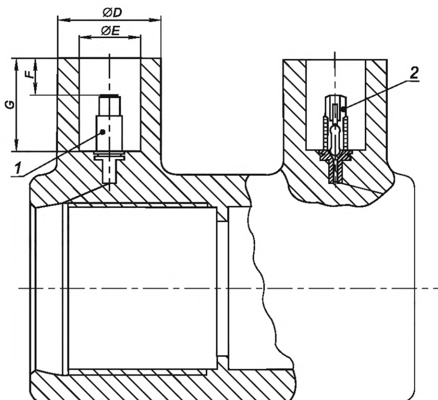
Рисунок D.1 — Вывод со встроенным резистором
