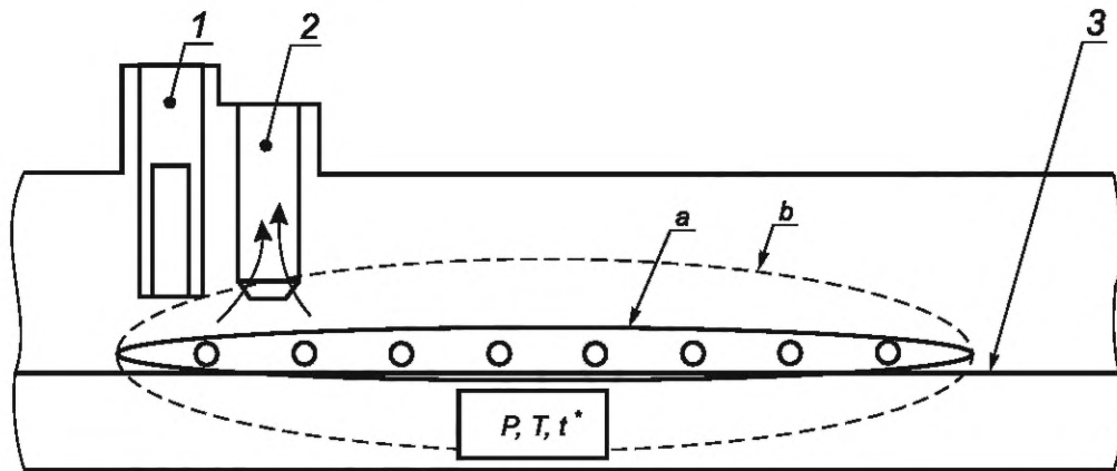
1 — вывод фитинга; 2 — канал; 3 — граница; а — граница зоны а (см. 4.3.3); б — граница зоны б (см. 4.3.3)
