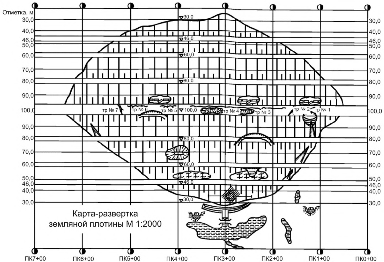
Рисунок А. 1 — Нанесение условными обозначениями данных визуальных натуральных наблюдений на масштабную карту-развертку грунтовой плотины (пример)
