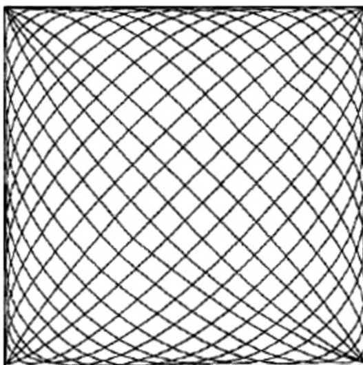
Рисунок 1 — Фигура Лиссажу
