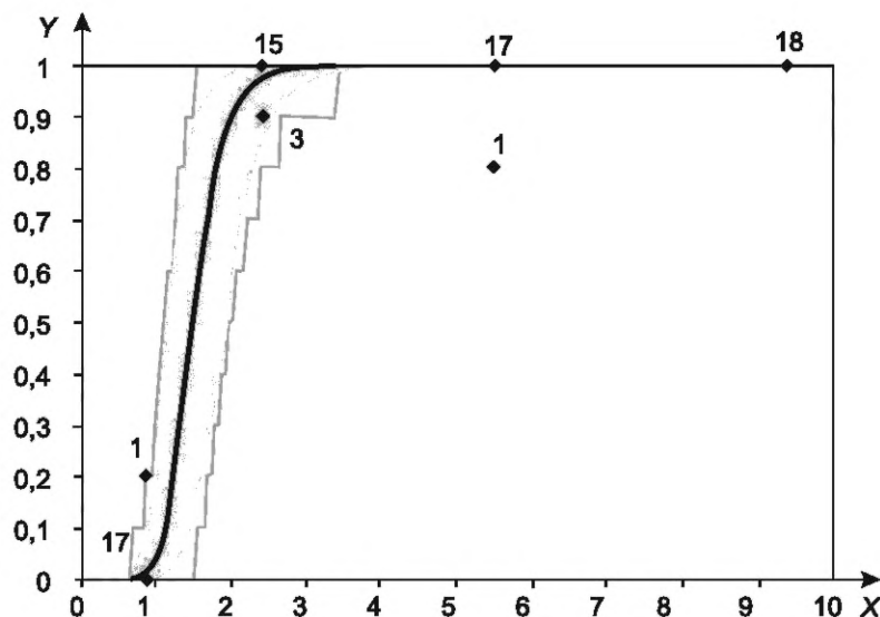
Рисунок 1 — Кривая средней POD, ROD конкретных лабораторий и предикционные интервалы
