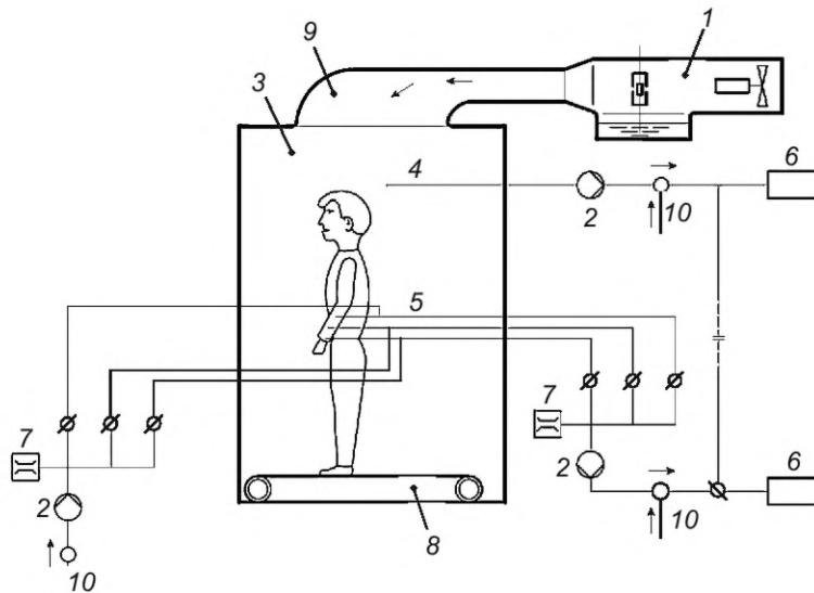
1 — распылитель; 2 — насос; 3 — камера; 4 — точка отбора проб из испытательной камеры; 5 — пробоотборные трубки к костюму (комбинезону) и от него (трубки для отбора проб и подачи воздуха); 6 — фотометр; 7 — расходомер; 8 — беговая дорожка; 9 — короб и дефлектор; 10 — дополнительная подача чистого сухого воздуха
