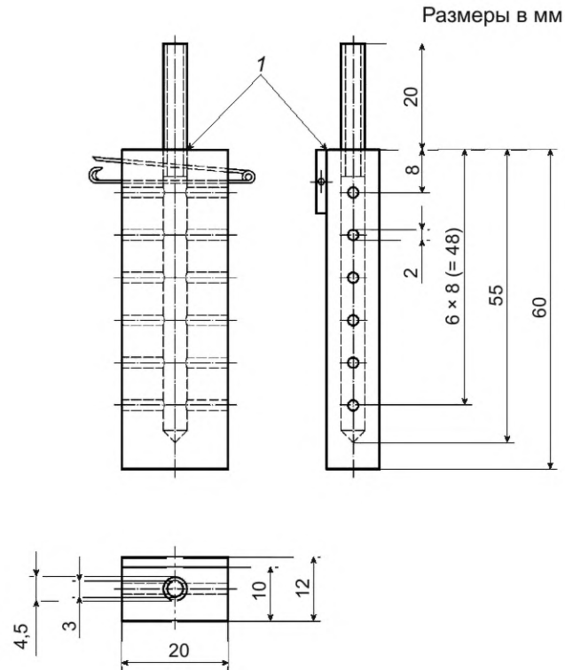
Рисунок 3 — Пробоотборник
