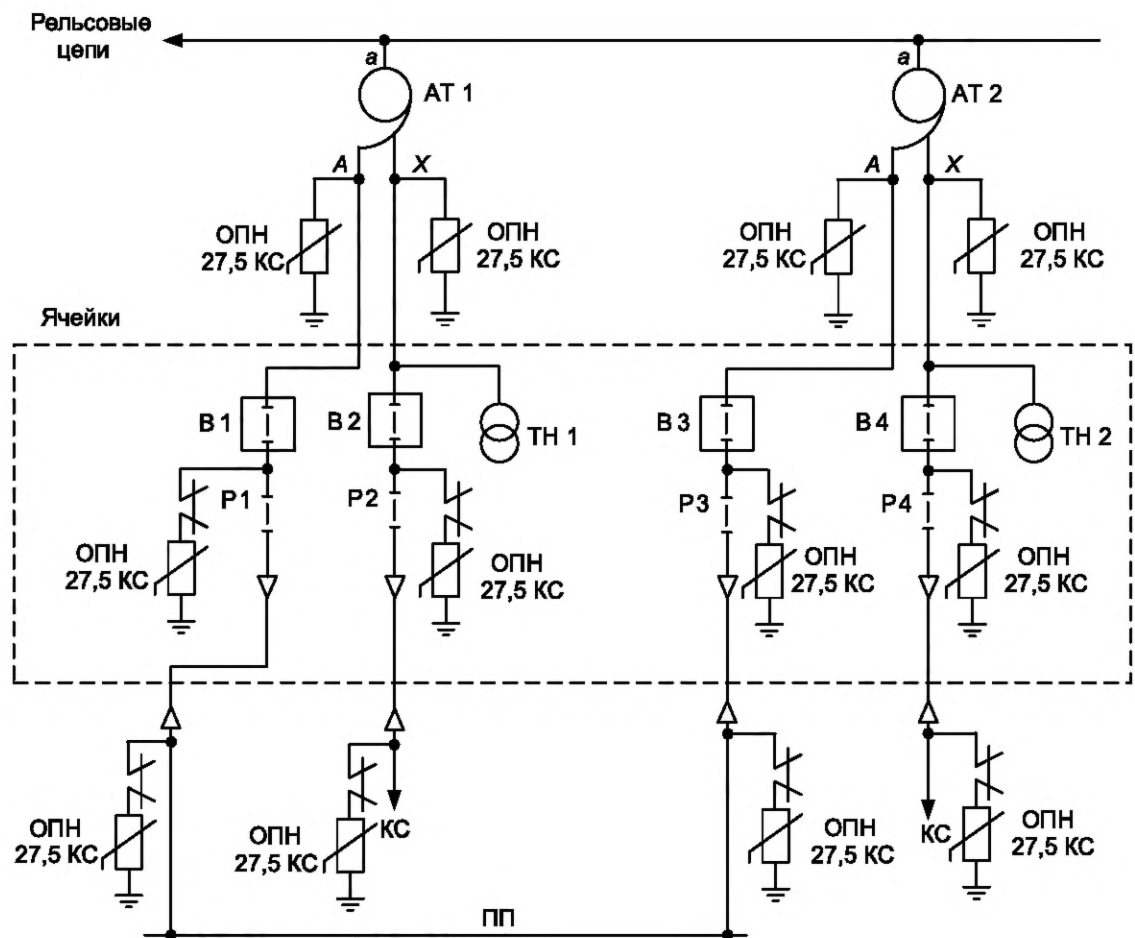
АТ 1, АТ 2 — автотрансформаторы; А, Х, а — выводы автотрансформатора; ТН1, ТН2 — трансформаторы напряжения; В1—В4 — выключатели; Р1—Р4 — разъединители; ПП — питающий провод
