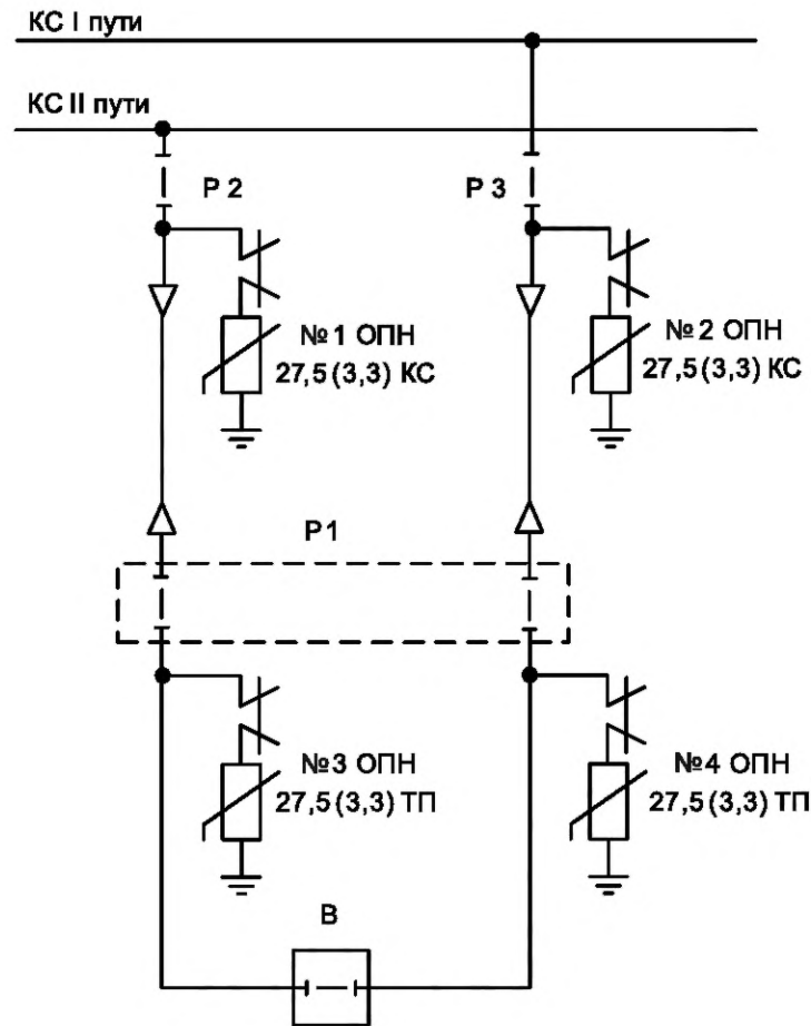
P1—P3 — разъединители; B — выключатель
