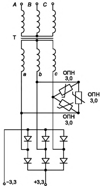
A, B, C, a, b, c — выводы трансформатора; T — силовой трансформатор
