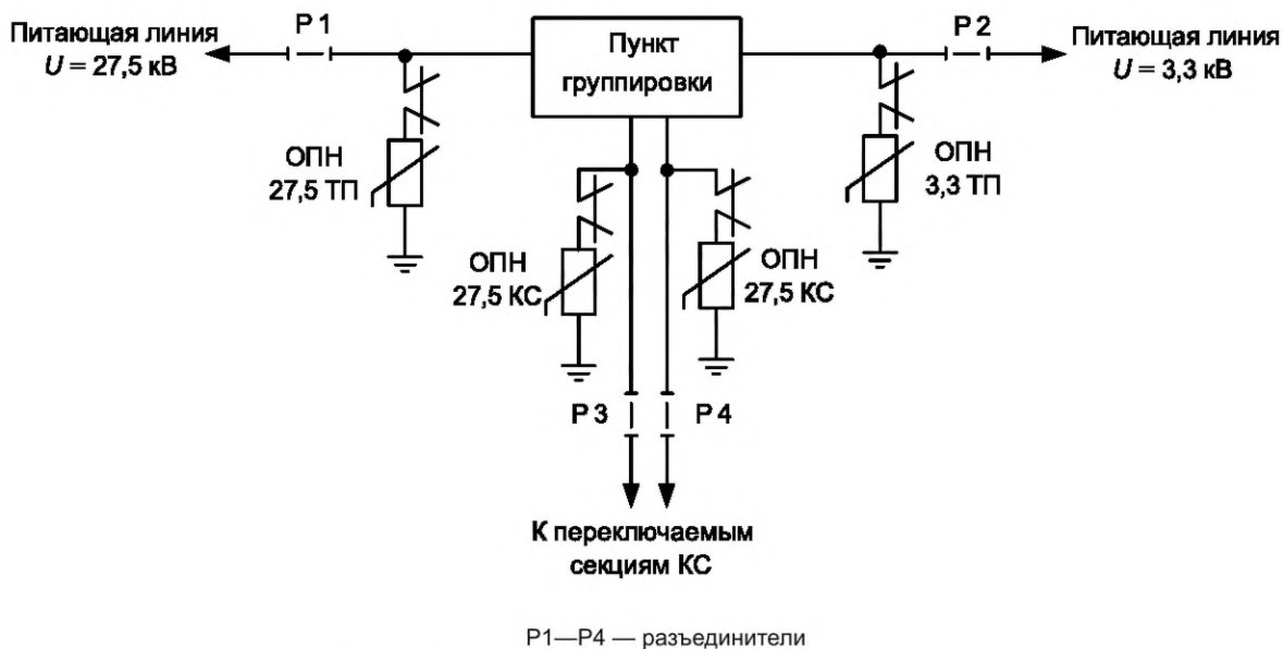
Рисунок 12 — Места установки ОПН на пункте группировки
