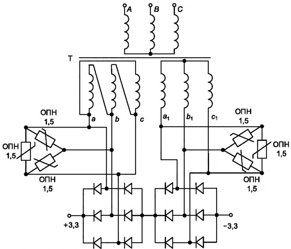
A, B, C, a, b, c, a 1 , b 1 , c 1 — выводы трансформатора; T — силовой трансформатор
