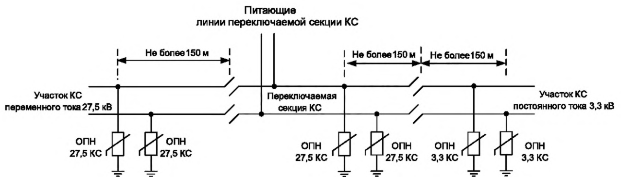
Рисунок 13 — Места установки ОПН на станции стыкования
