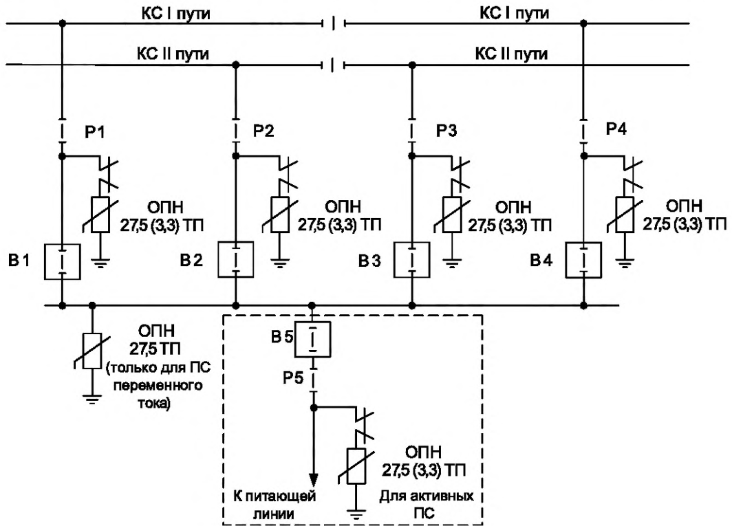
P1—P5 — разъединители; B1—B5 — выключатели
