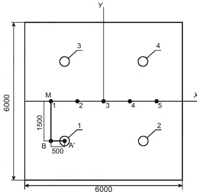
Рисунок Б.3 — Расположение световодов в помещении
